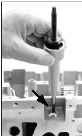
Remoção da vela de incandescência
