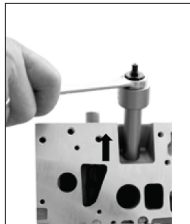
Vela incandescente removida
