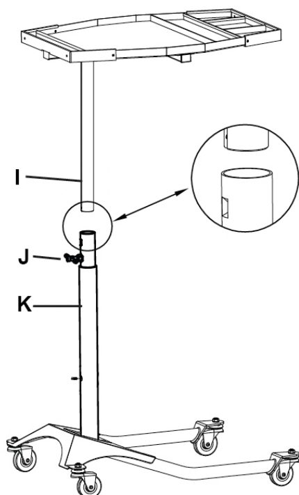
Figura 4 - Fixação das Colunas
