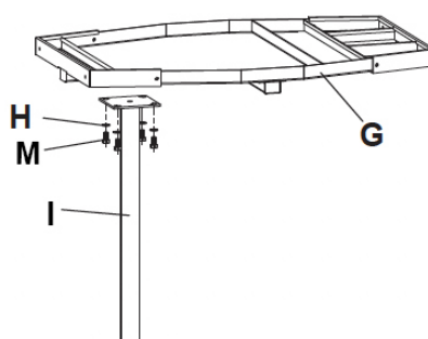
Figura 2 - Fixação da Coluna à Bandeja
