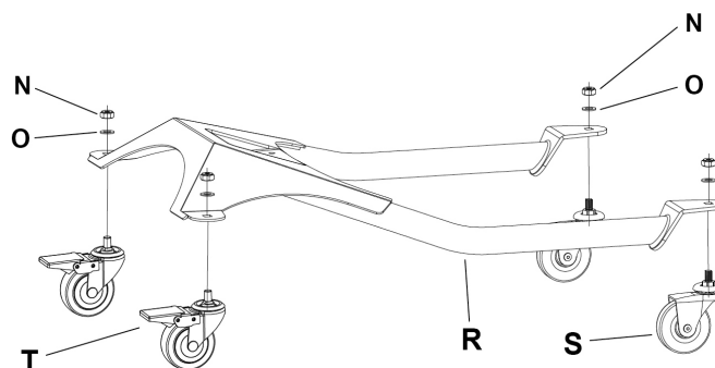
Figura 1 - Montagem da Base
