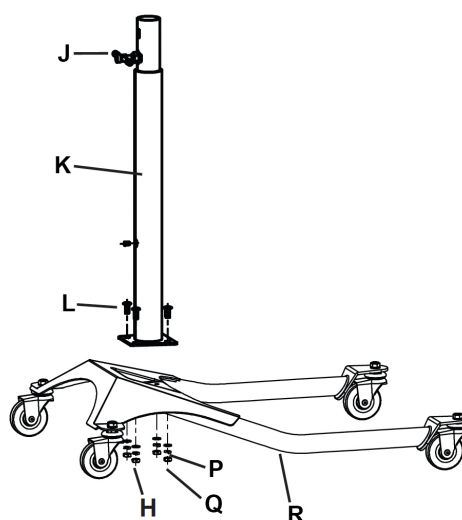
Figura 3 - Fixação da Coluna à Base
