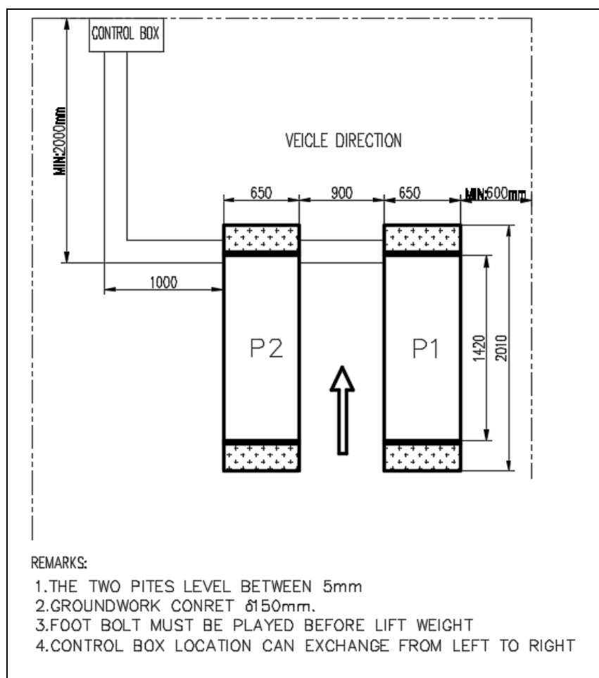
Figura 4 (Esquema)
