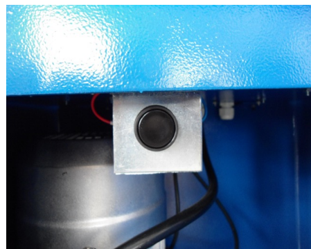
Figura 18 botão de ajuste de nível (SB4)
